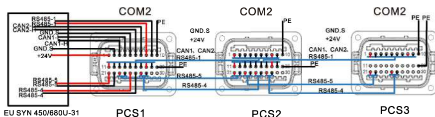
Schéma paralelního zapojení (tři zařízení)
