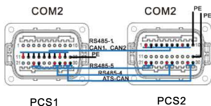
Schéma zapojení paralelních (dvou zařízení)
