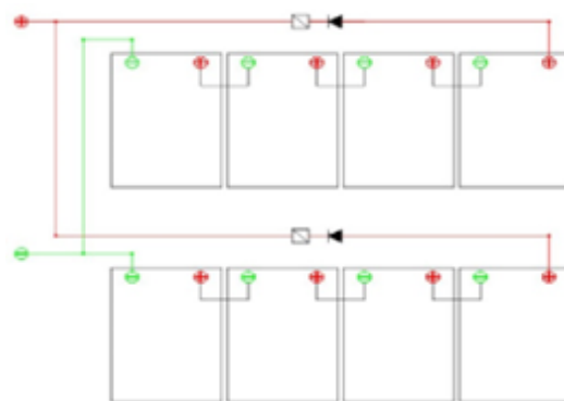
Paralelní zapojení po sériovém zapojení
