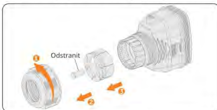
Obrázek 8-43 Rozebrání konektoru
