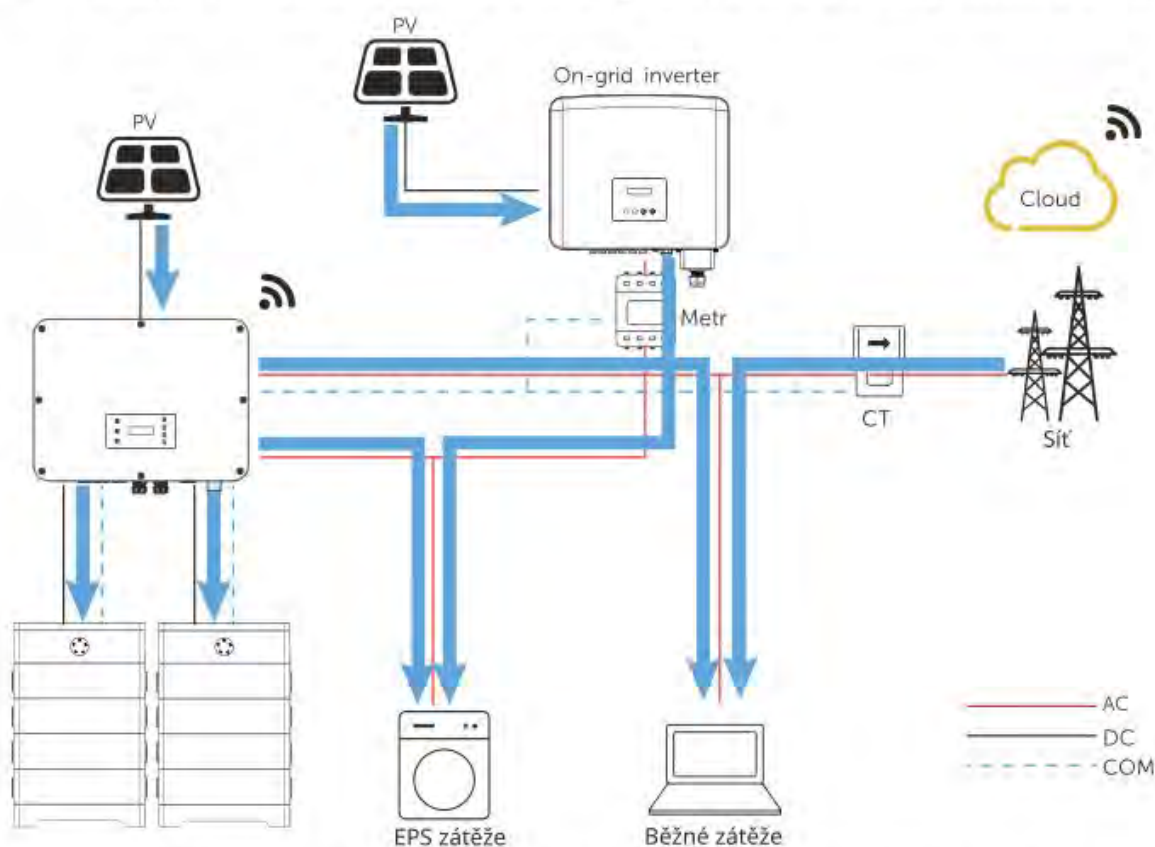
Obrázek 15-14 Tok energie, když je sít' zapnuta a PV dostatečné
