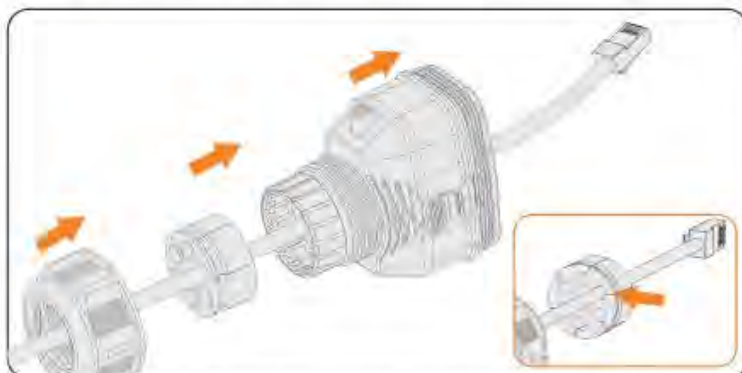
Obrázek 8-44 Provlékání kabelů
