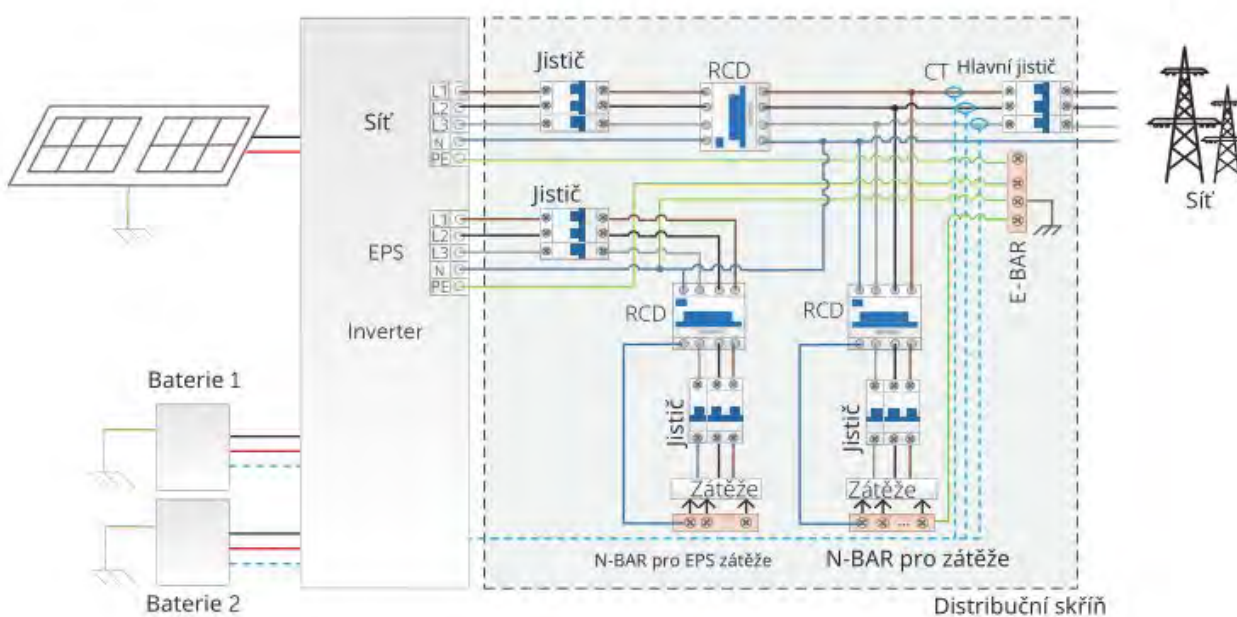
Obrázek 2-9 Částečná záloha domácnosti pro Austrálii
