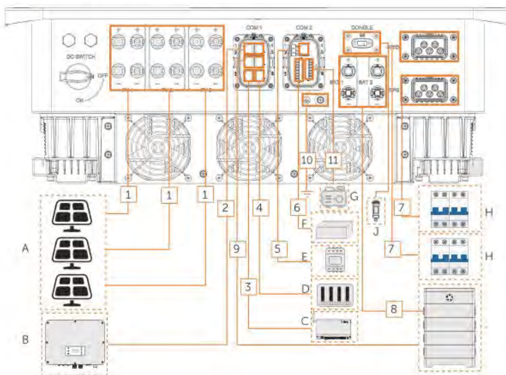
Obrázek 8-2 Kabelová připojení inverteru
