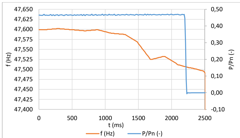
Obr.12.10: Podfrekvenční ochrana
