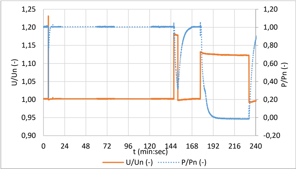
Obr.10.2: Křivka ORVT
