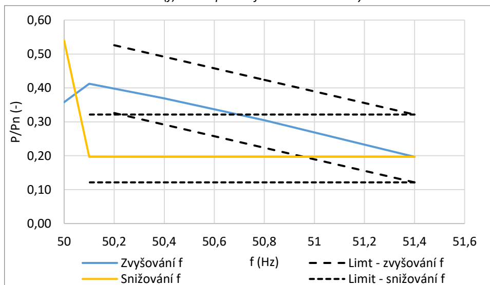
Obr.3.3: P(f) křivka při nadfrekvenci – 37 % výkonu
